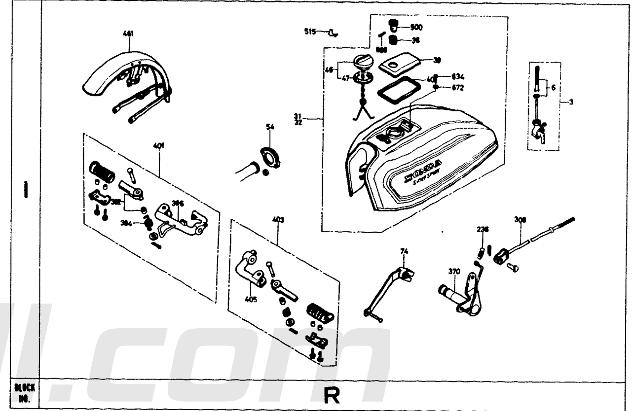
CB400F2-A TYPE
